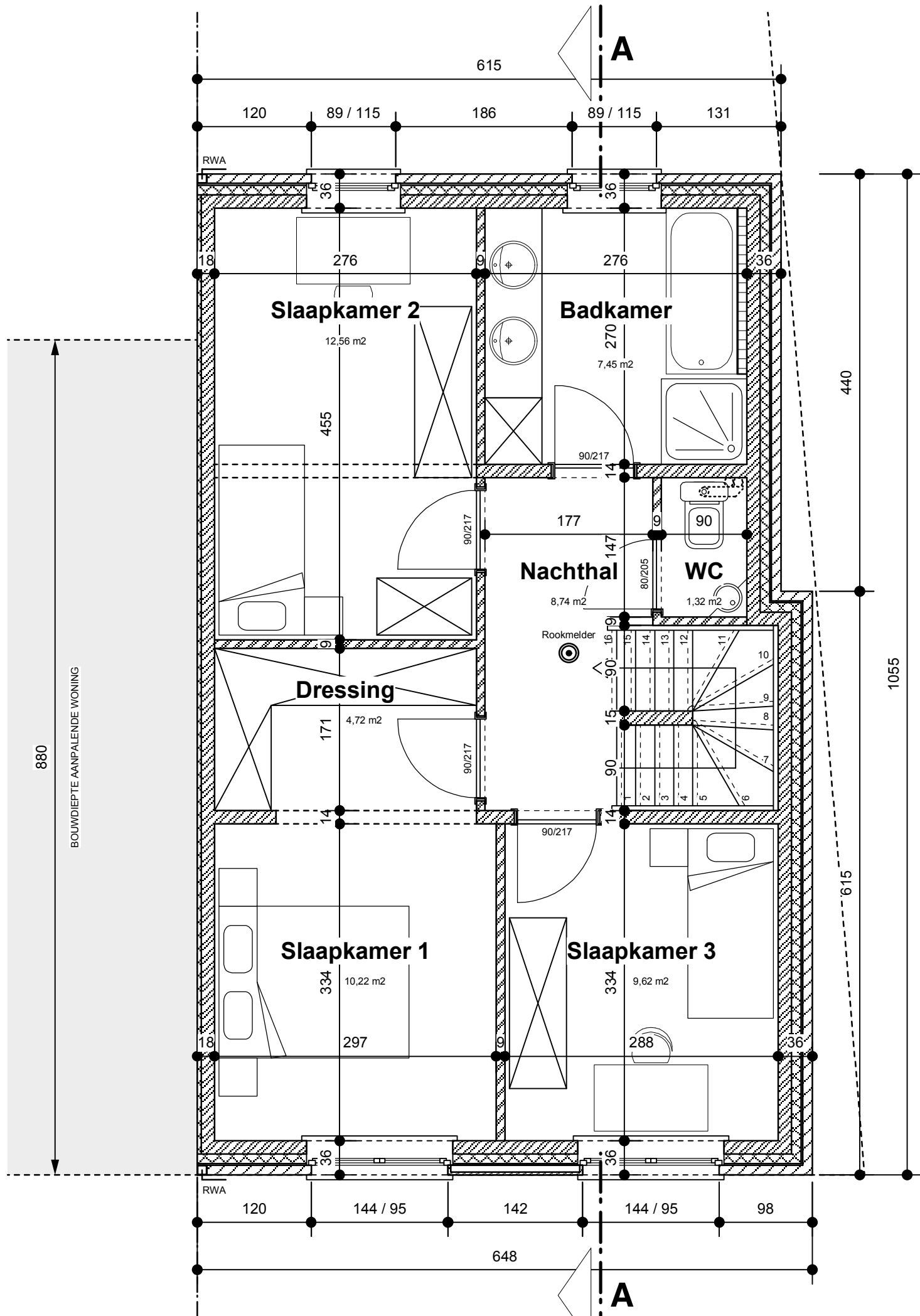
VERDIEPINGSPLAN - Schaal 1/50
