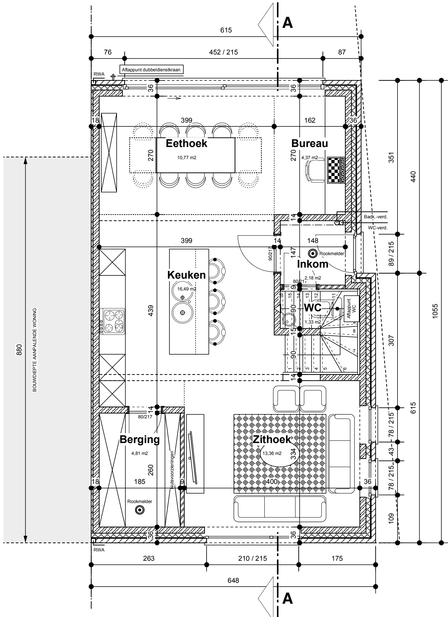
GRONDPLAN - Schaal 1/50
